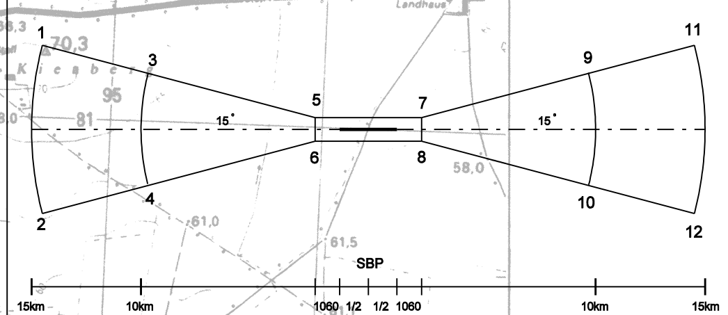
Start- und Landebahn Sicherheitsflächen und Anflugsektoren nach § 12 LuftVG
